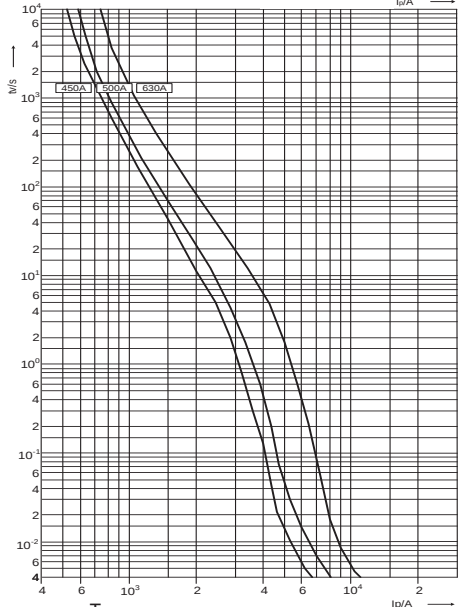
Токо-временные характеристики ножевых предохранителей NH gPV, PV (gR) 1100 VDC
