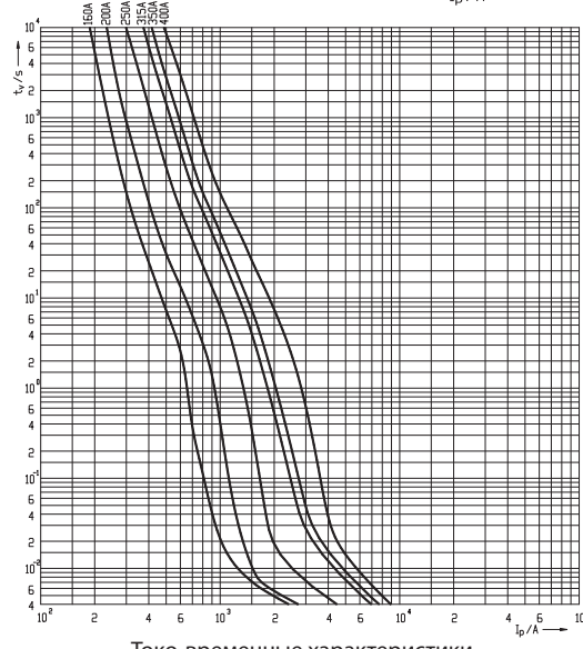
Токо-временные характеристики ножевых предохранителей NH gPV 1000 VDC
